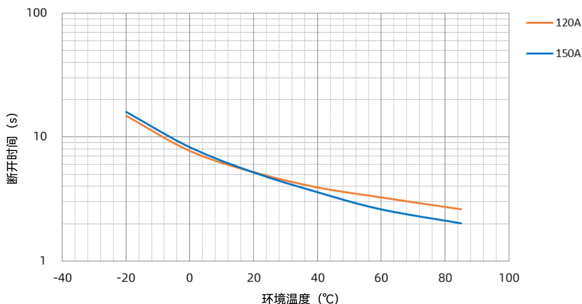
SKT 温度-时间曲线
