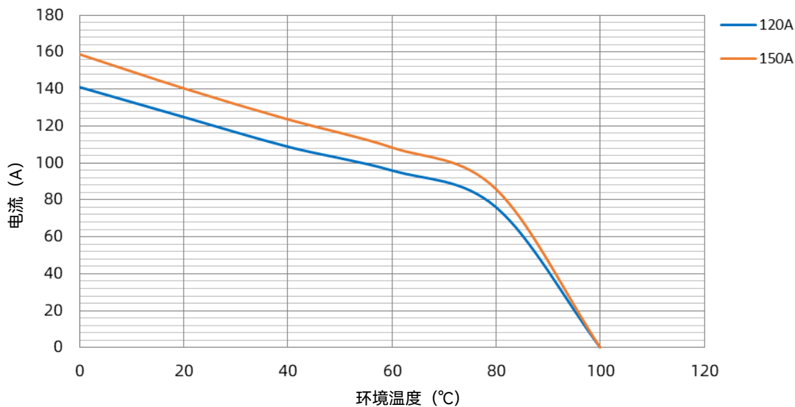
SKT 载流能力曲线
