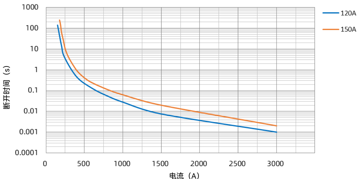
SKT 电流-时间曲线
