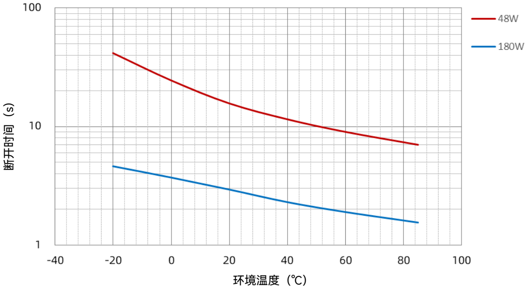
SKT 150 A 功率-温度曲线
