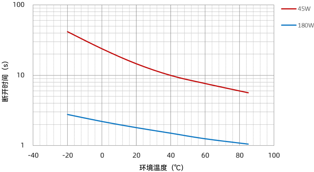
SKT 120 A 功率-温度曲线
