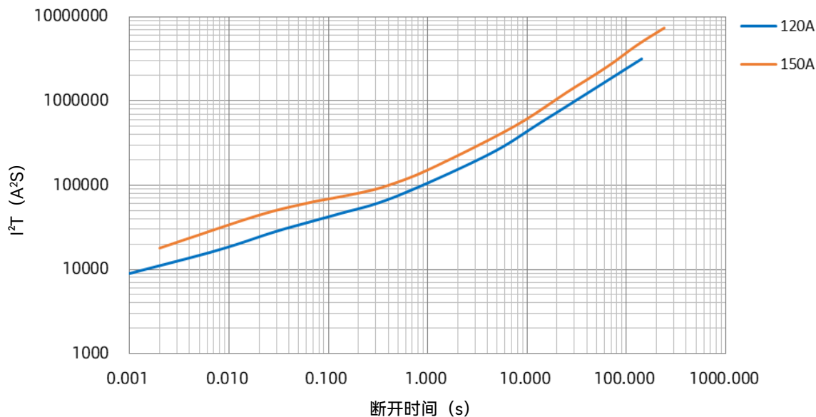
SKT I²t-t 曲线
